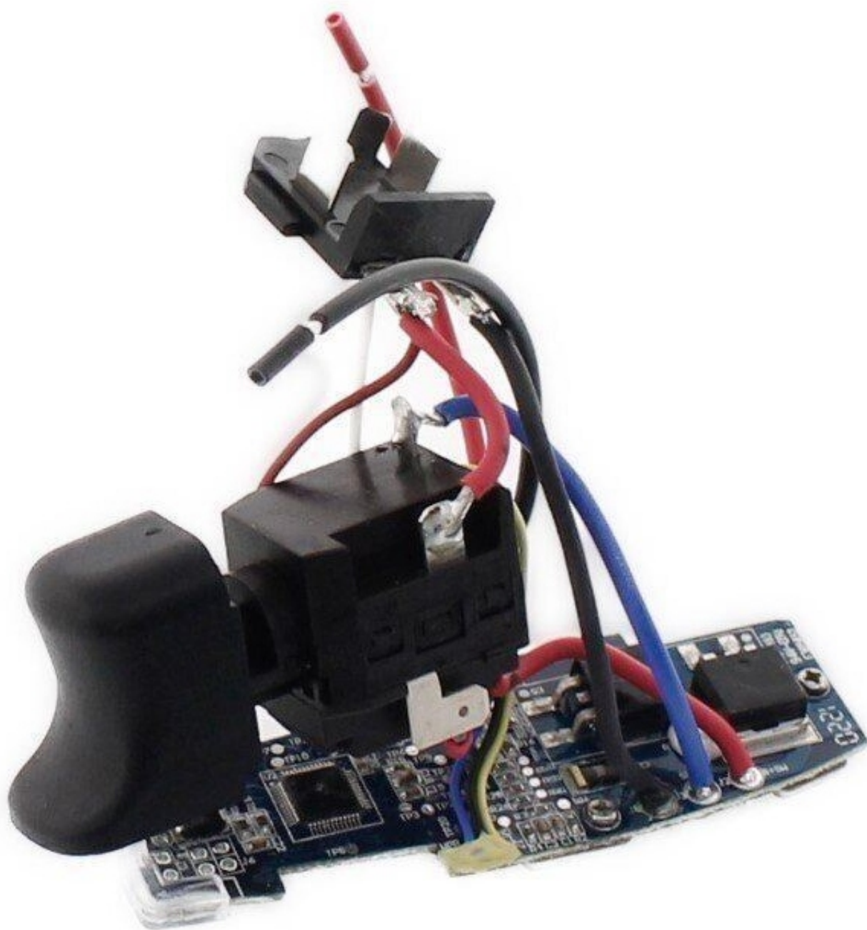
Wyłącznik do wkrętarek Milwaukee M12BD, M12BDD, M12BPD, M12BDDX
